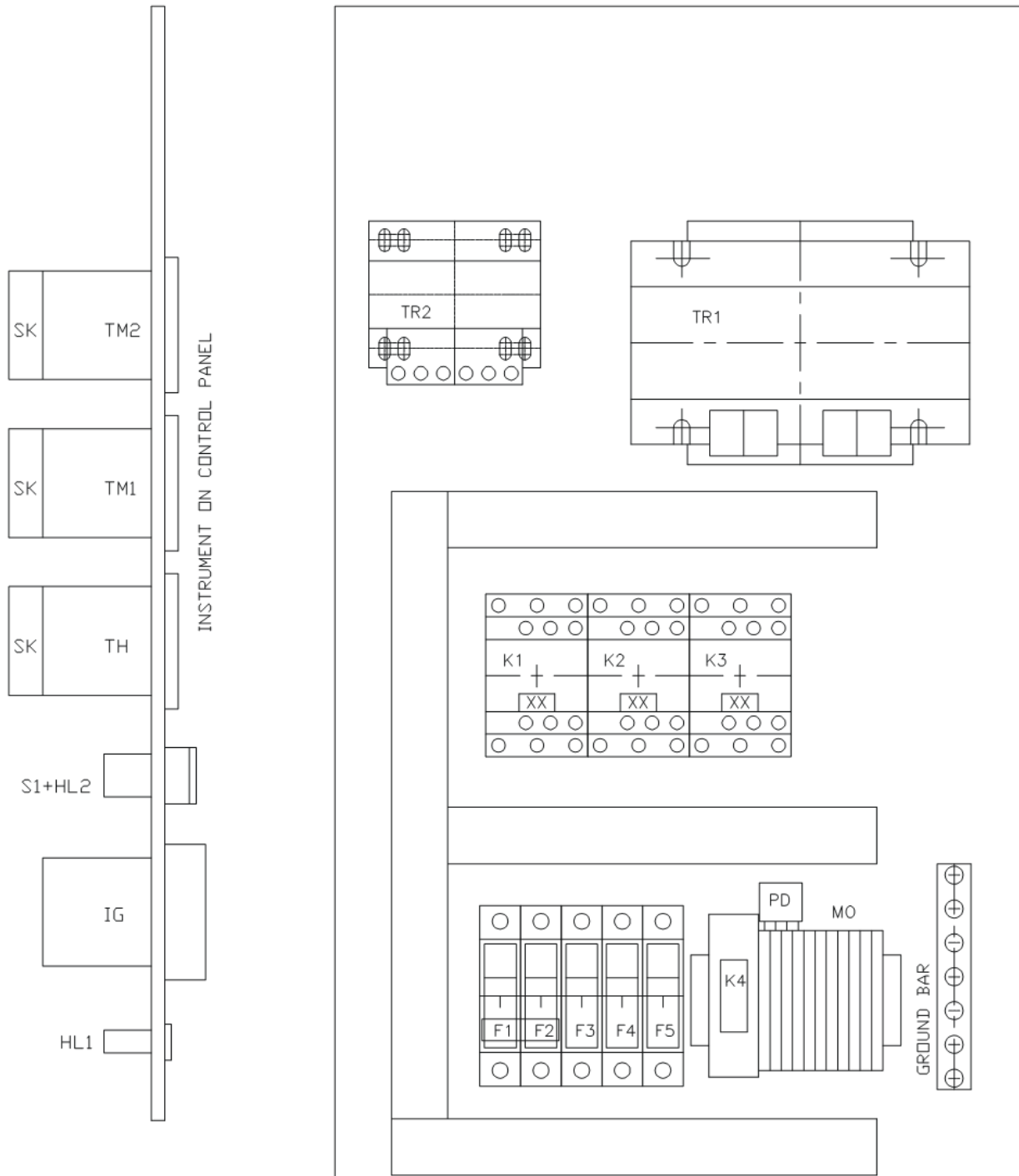
PIANTA COMPONENTI ELETTRICI IMPIANTO 3246-4255 STCN LAY-OUT ELECTRICAL COMPONENTS 3246-4255 STCN
